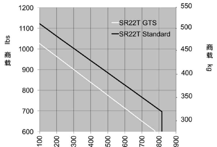
SR22T 高速巡航@8,000英尺 (180KTAS)
