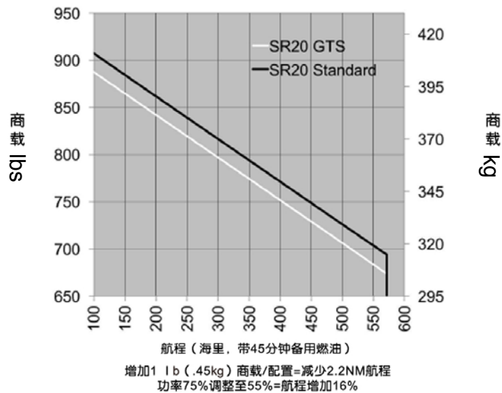
SR20 高速巡航@8,000英尺 (155KTAS)
